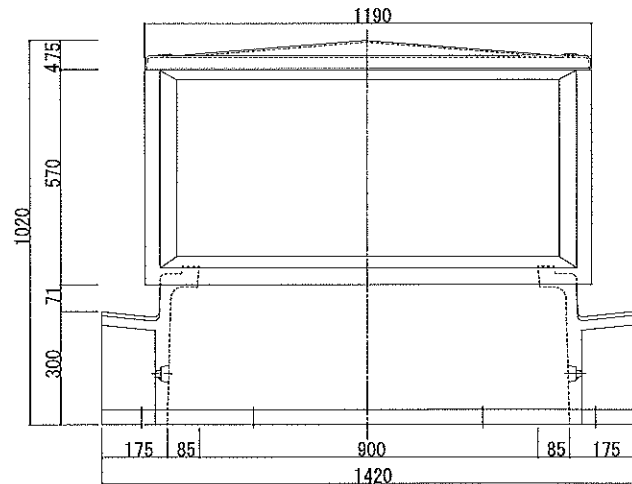
立面図
